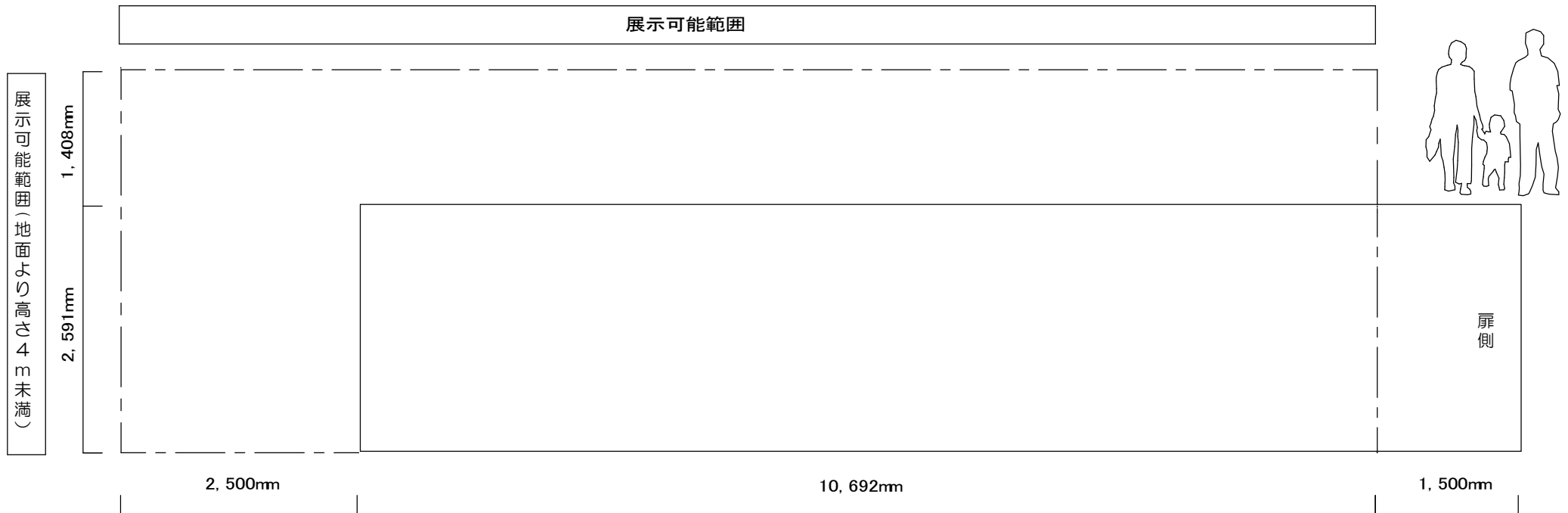
側面図 縮尺 1/60
