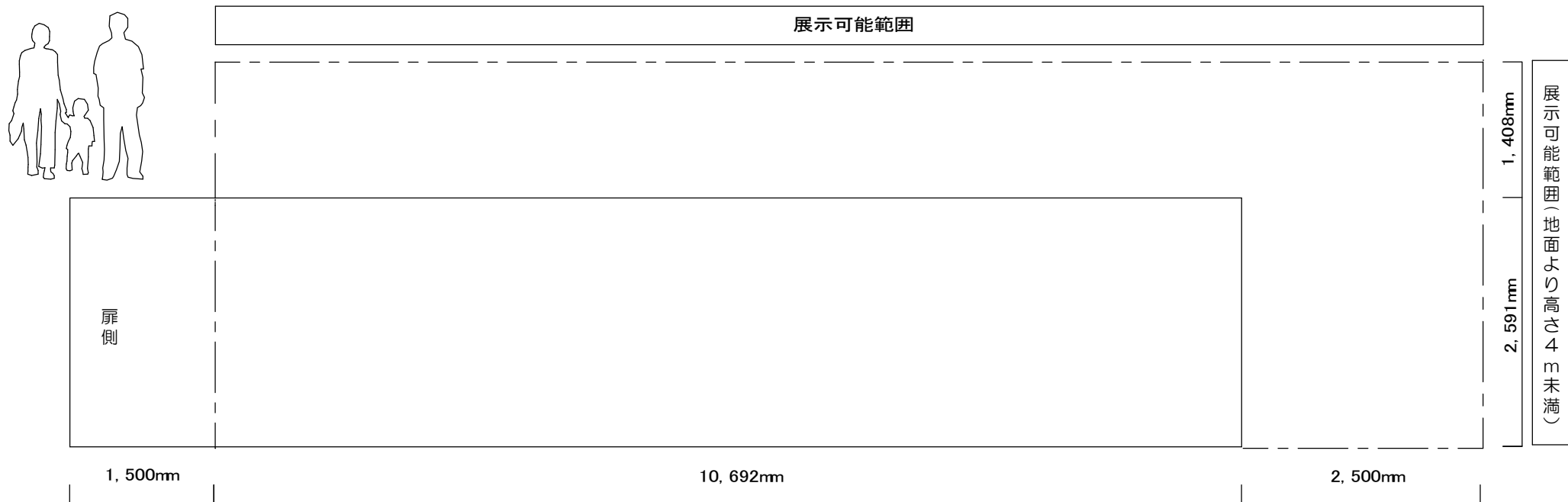
側面図 縮尺 1/60
